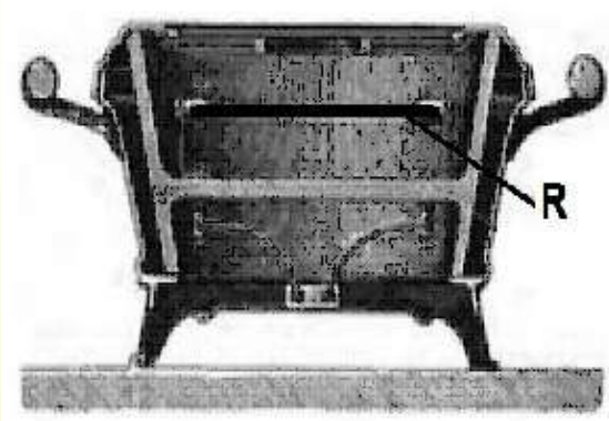
1899 Elemento calefactor cerámico metálico de Parvillée (documento del Museo Ultimheat)
